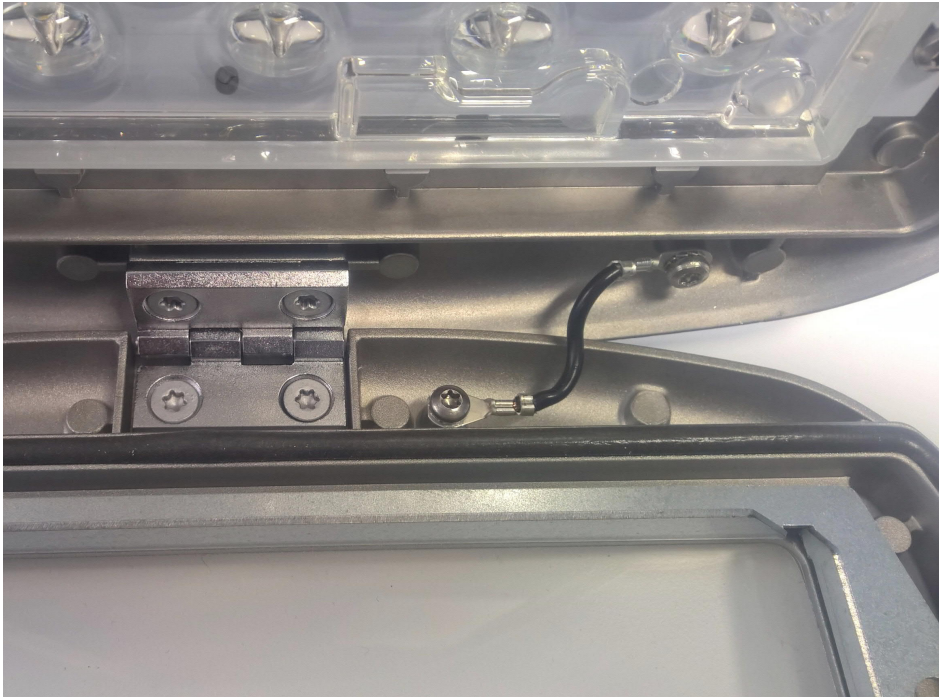
Kuva 1. Valaisimen runko-osien välinen maadoitusjohdin.
